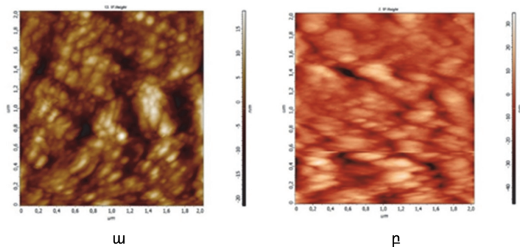
Նկ. 2. Գազային խառնուրդում ազոտի փարբեր քանակների և իոնային աղբյուրի 120 Վտ հզորության դեպքում ստացված նմուշների ափոմա-ուժային մանրադիփակով ստացված պարկերները. ա- 10%; բ- 20%
