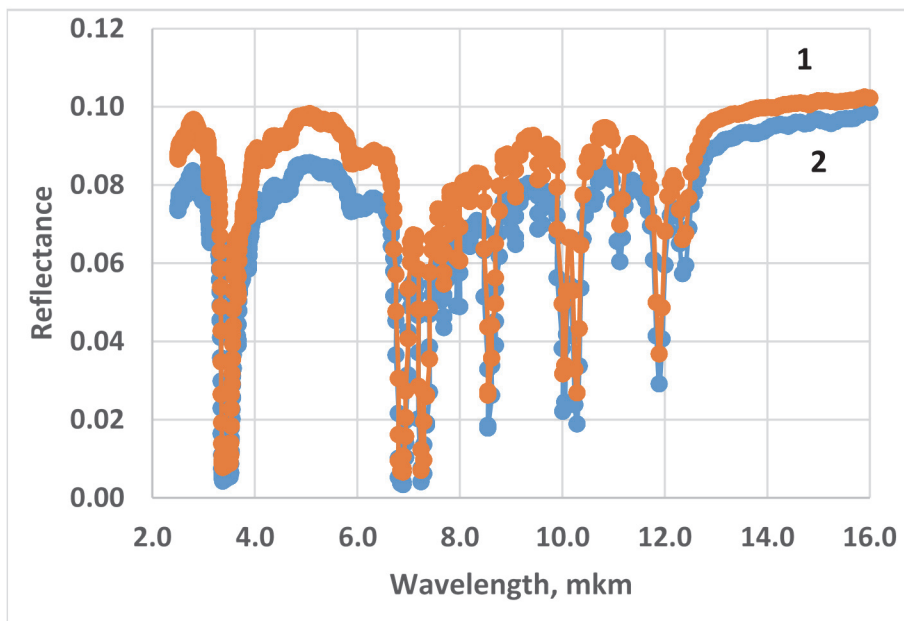
Նկ. 3. Անդրադարձման սպեկտրալ գործակիցները՝ ա- 0.2-1.1 մկմ և բ- 2.0-16.0 մկմ հատվածում իոնային աղբյուրի 120 Վտ հզորության և գազային խառնուրդում ազդեցիկ տարրեր քանակների դեպքում. 1- N=5%; 2- N=20%
